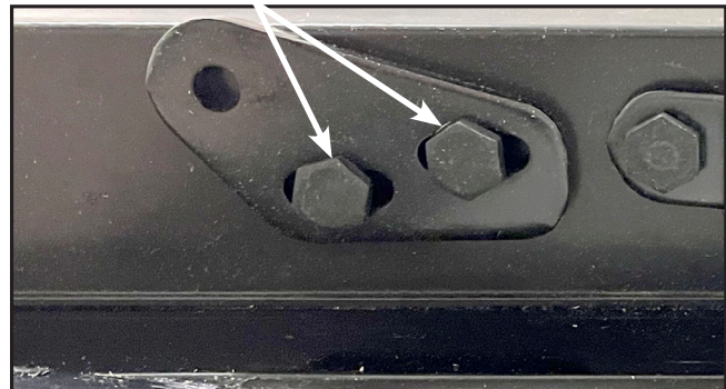
Adjust Door Sag
